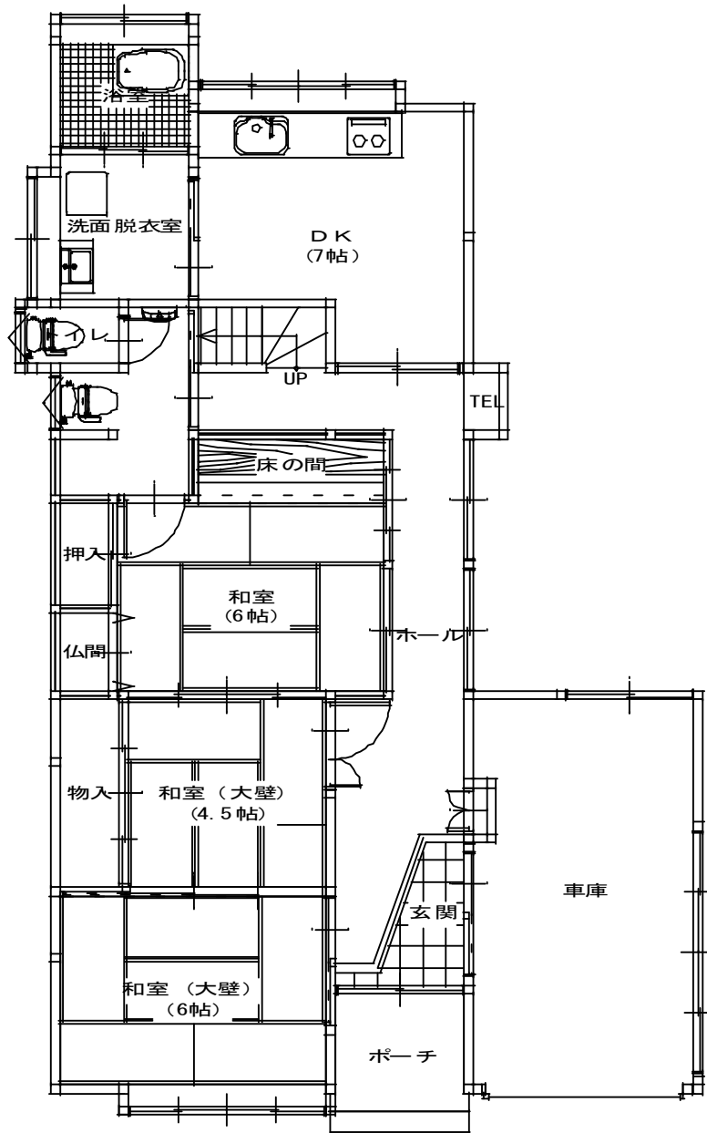
1階平面図
