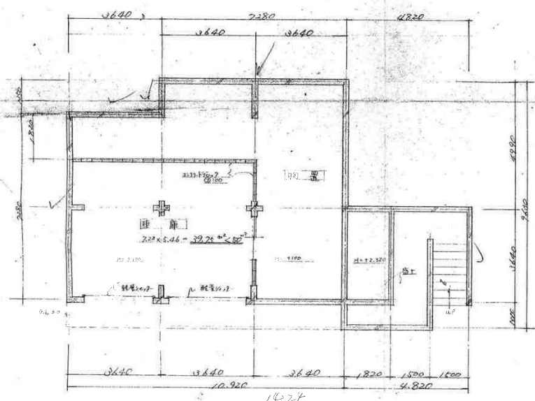
1階平面図 1/100
