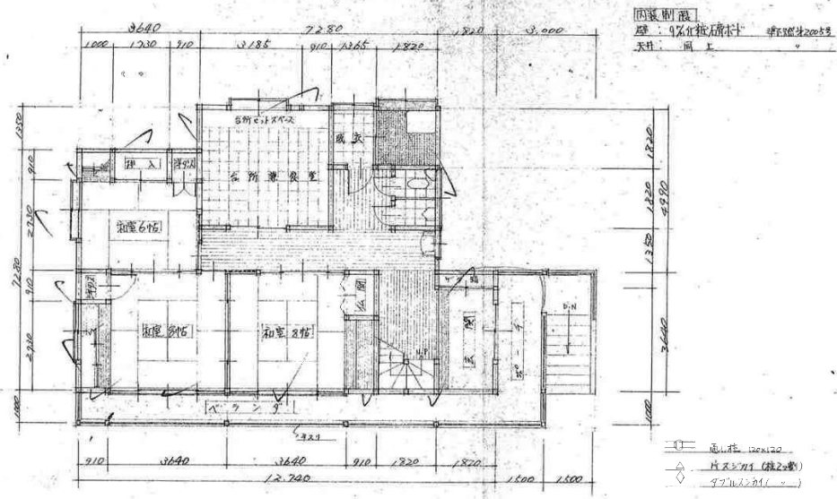
2階平面図 1/100
