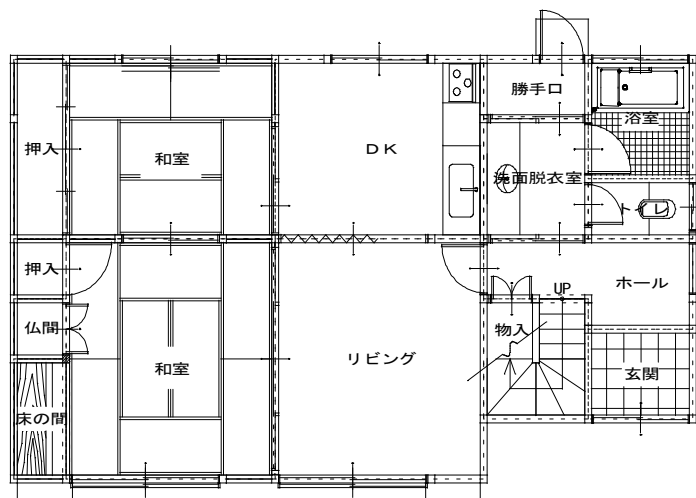
1 階平面図
