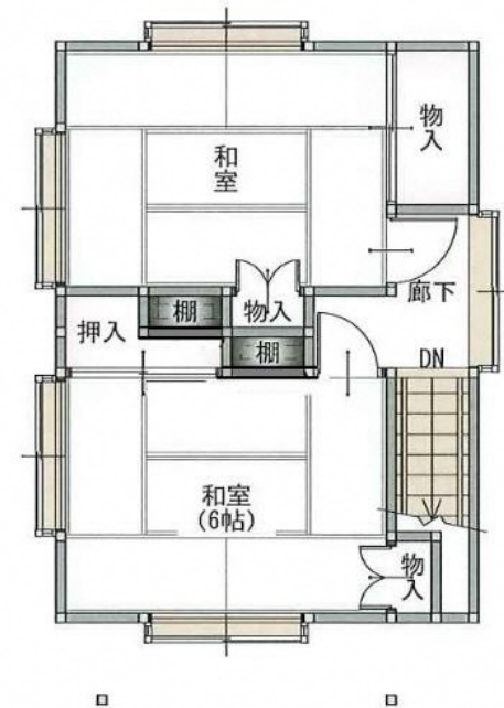
2階 平面図 S:1/100
