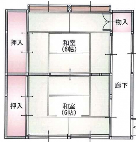
2階 平面図 S:1/100
