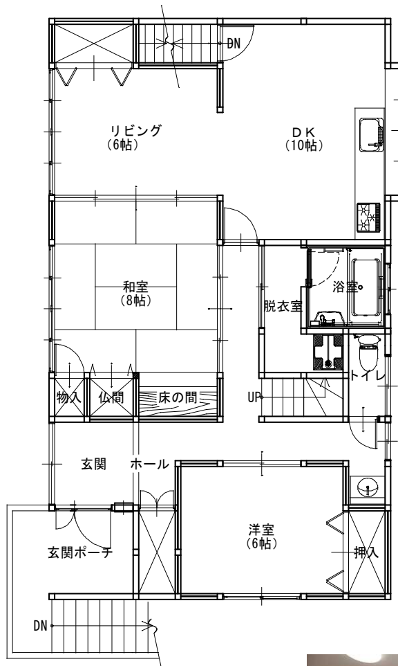
1 F 平面図
