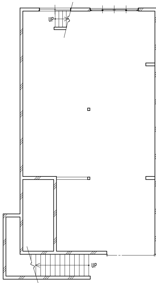
床下部分平面図
