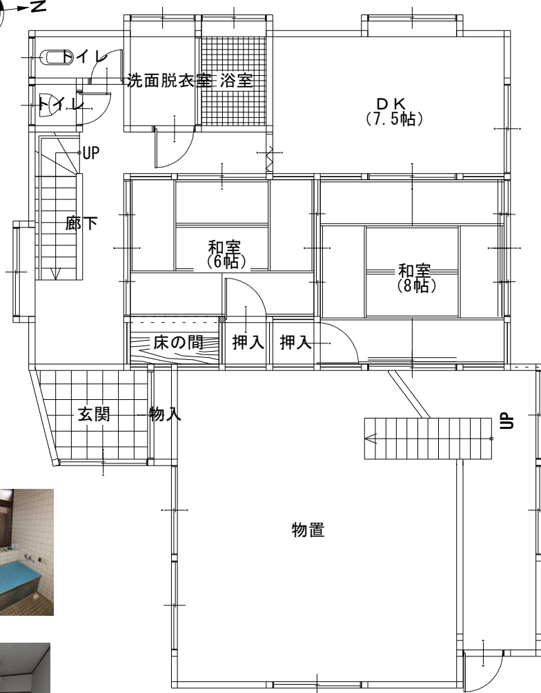
1階平面図
