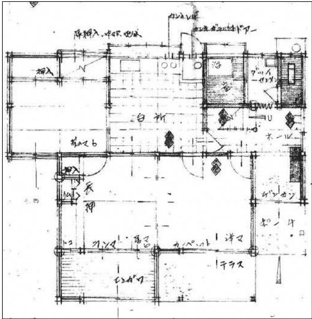
▲ 1階
